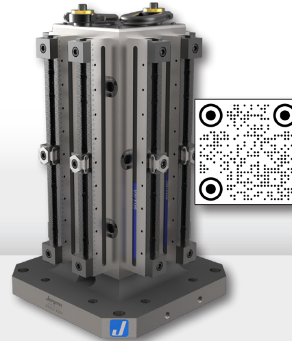
OK-VISE
